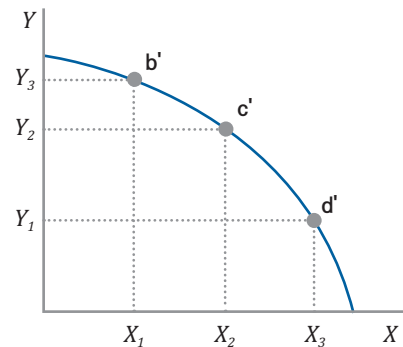
〈그림2-4〉 생산가능곡선
