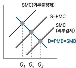
(b) 생산외부성
