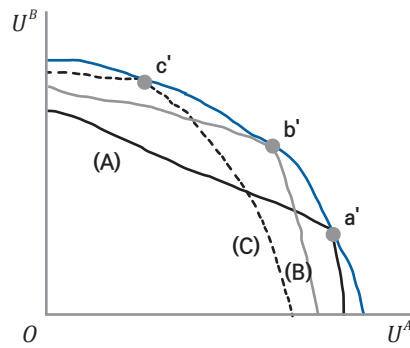
〈그림2-7〉 효용가능경계
