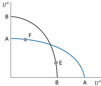
〈그림2-9〉 스키토프스키기준
