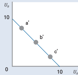
(b) 효용가능곡선
