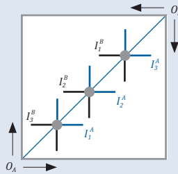
(a) 계약곡선
