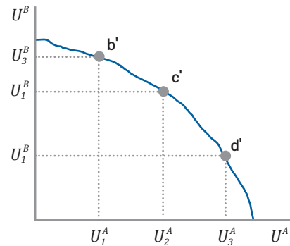
〈그림2-2〉 효용가능곡선
