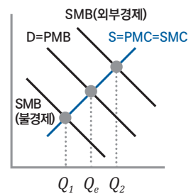
(c) 소비외부성
